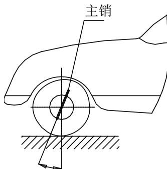
图1.4 主销后倾角示意图
